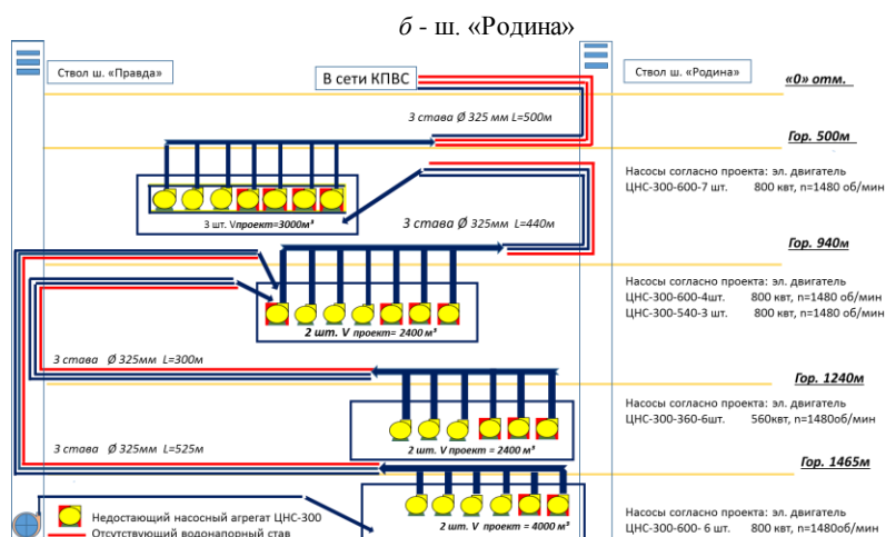
Рис. 3. Схемы водоотлива шахтных вод
