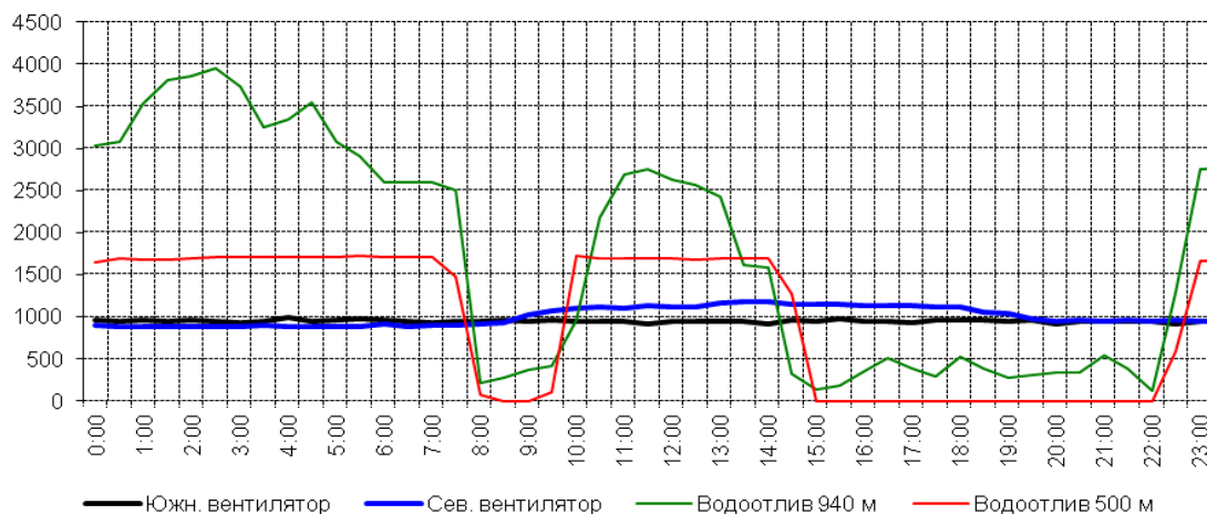
Рис. 1. Уровни суточного потребления электрической энергии отдельными энергоемкими подземными потребителями ш. Родина (г. Кривой Рог)
